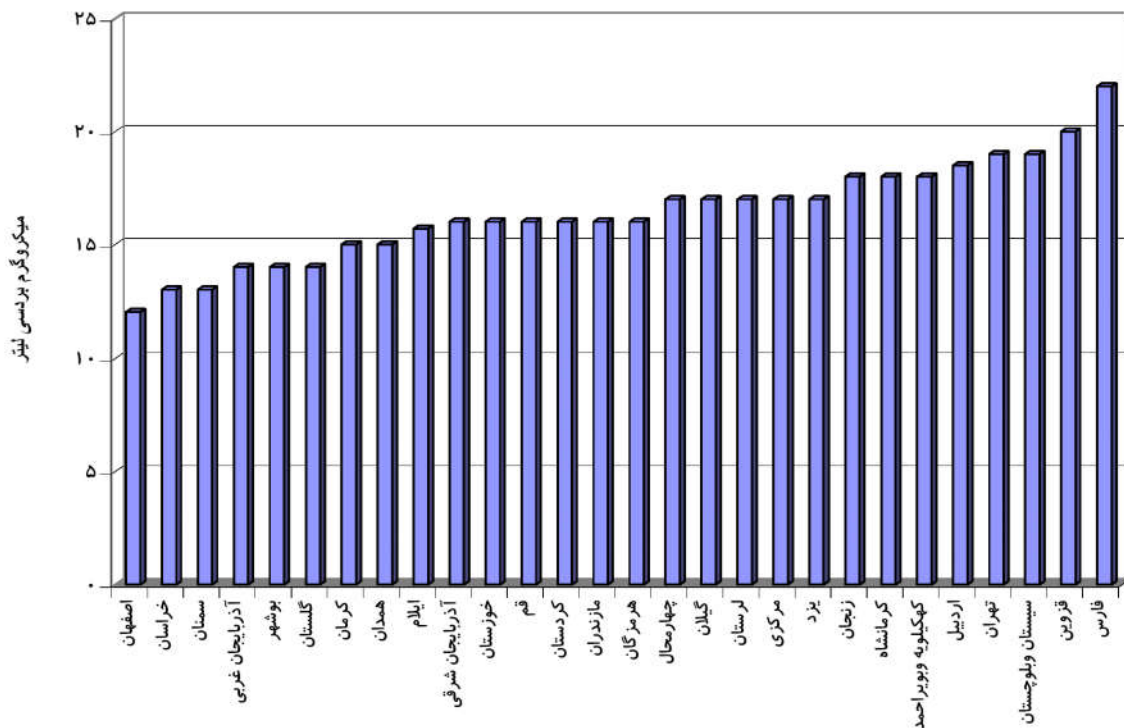
نمودار ۵ - میانگین عدد دانش آموزان ۱۰-۸ ساله استان‌های کشور (بررسی ملی سال ۱۳۸۰)
